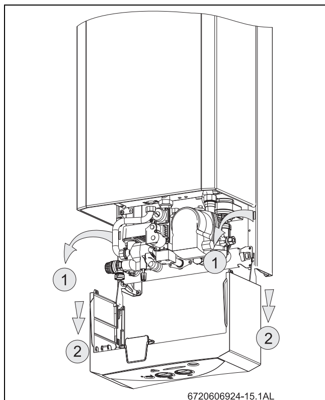
Fig. 28 Position de réglage pour accéder à l'électronique et de l'hydraulique
