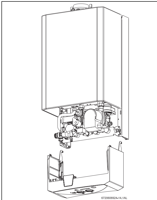
Fig. 11 Enlever le tableau électrique
