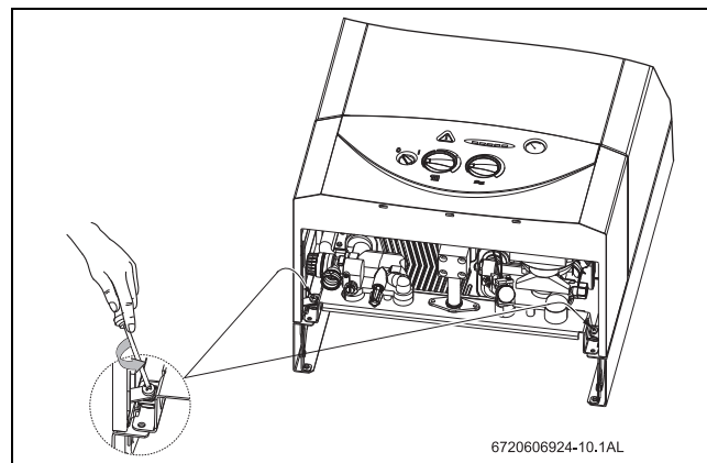
Fig. 9 Vis de sécurité
